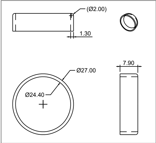
INSERT 1:1 SCALE
