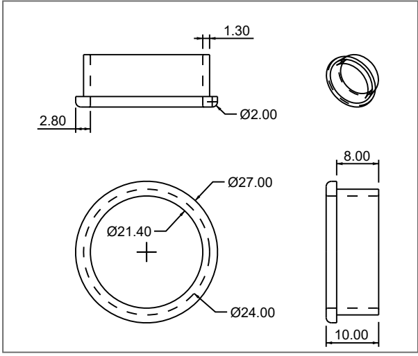
BASE 1:1 SCALE
